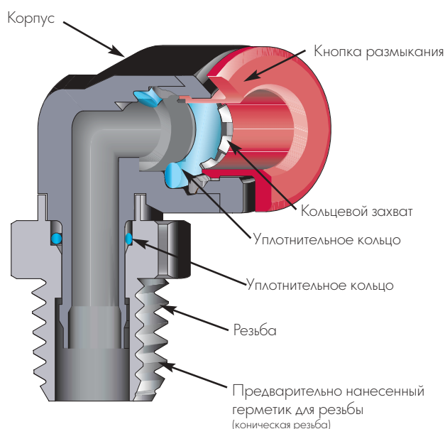
Типовой номер детали: C01470628 Коленчатый переходник с углом поворота 90°
